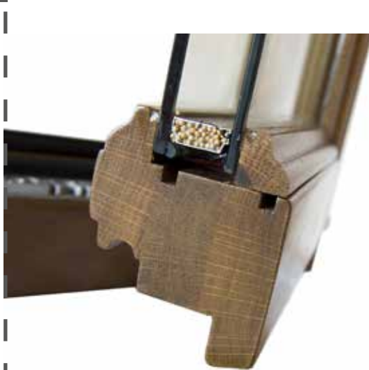
VISTA SEZIONE ANTA SASH SECTION
